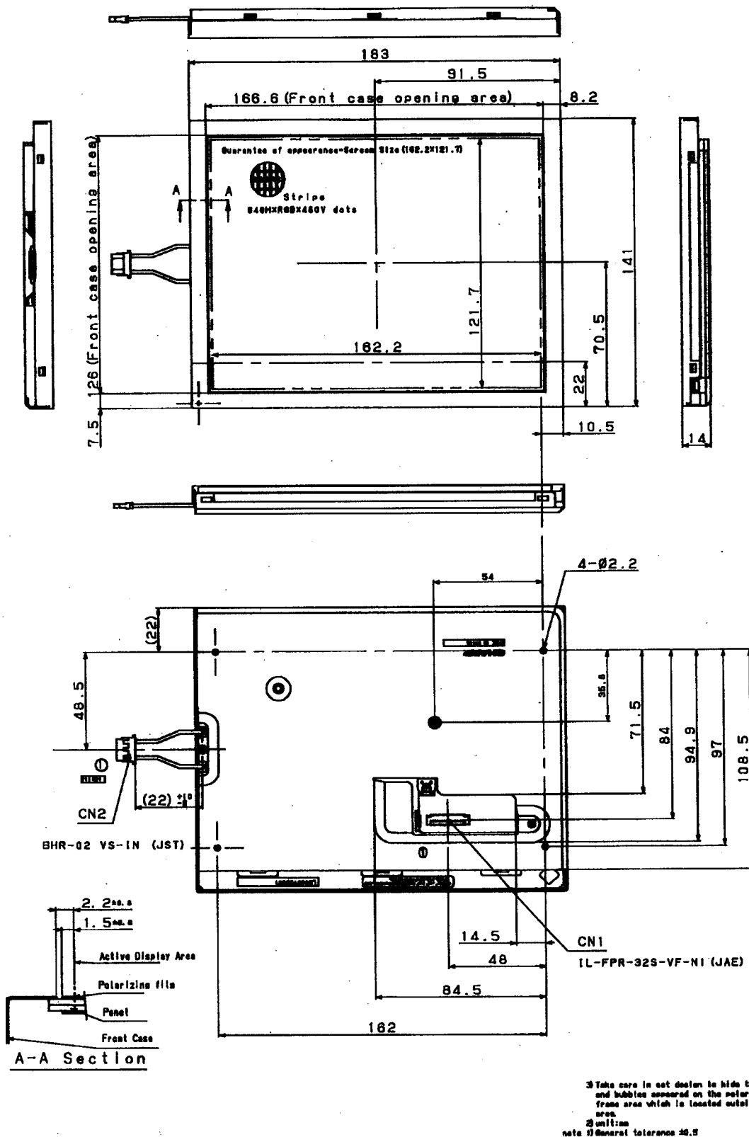
Fig.1 Module dimension
