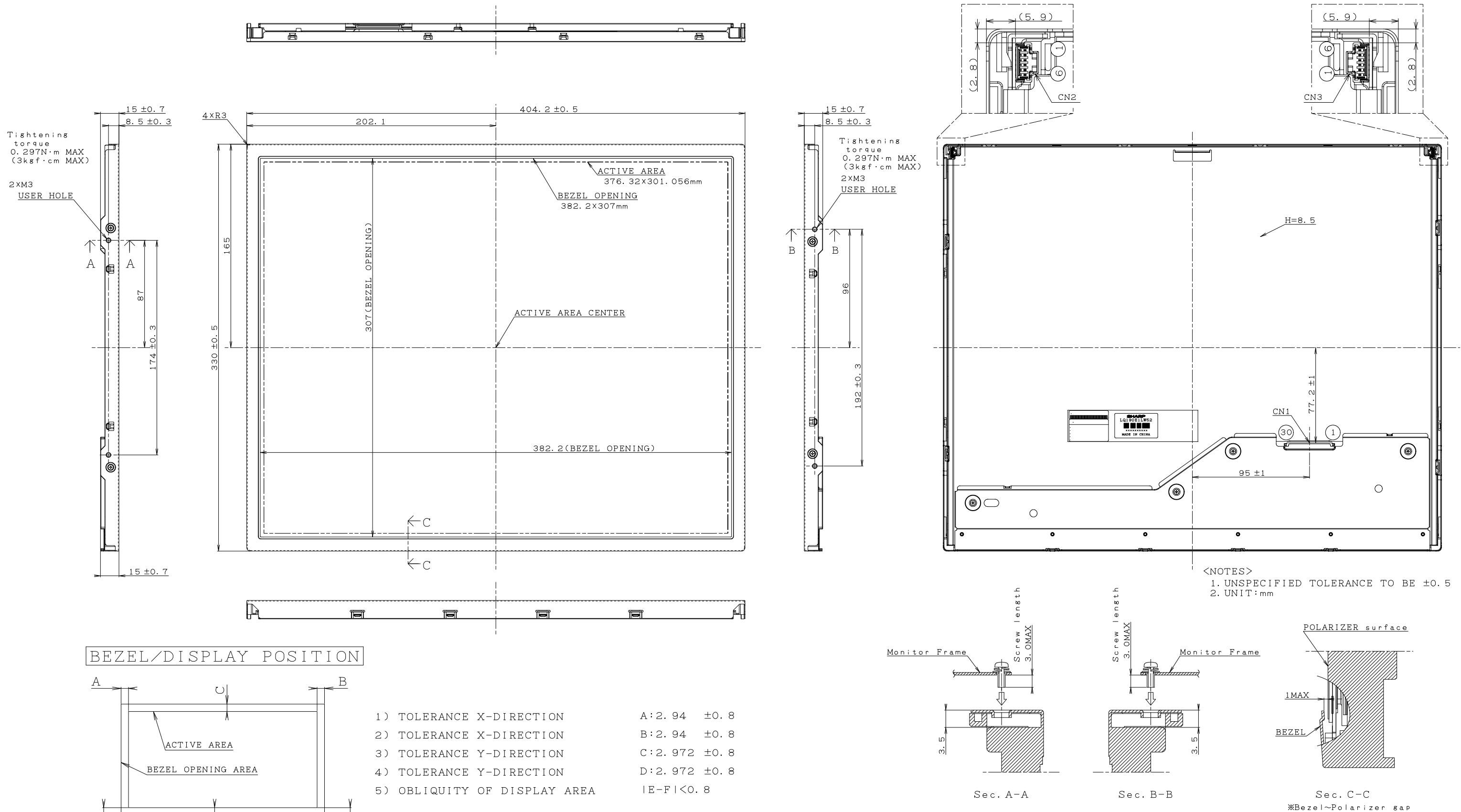
Fig. 1 Outline dimensions (LQ190E1LW52)
