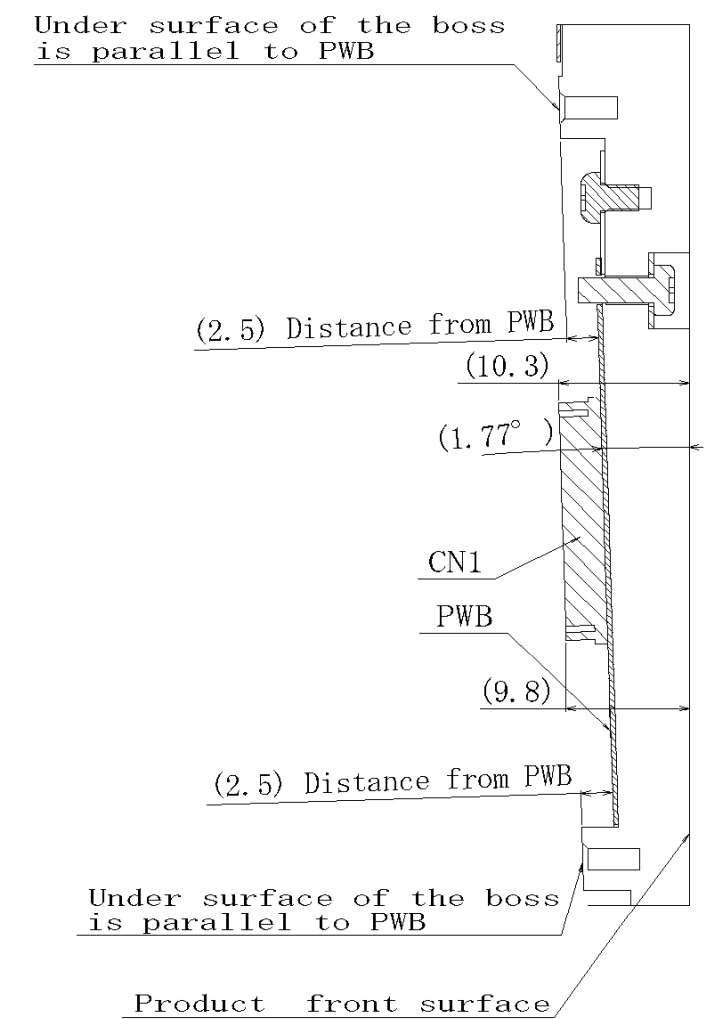
Sec. A-A
