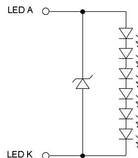
【LED Circuit (LED 回路)】
